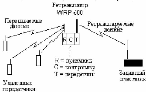
Рисунок 1 Конфигурация передачи сигналов
