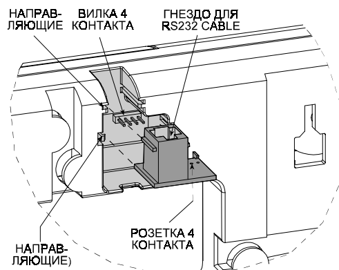
Рисунок 28. Установка модуля RS-232
