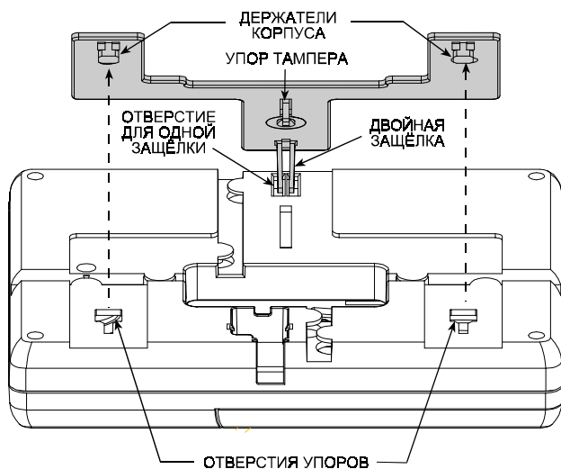
Рисунок 11. Соединение кронштейна и корпуса - Вид сверху
