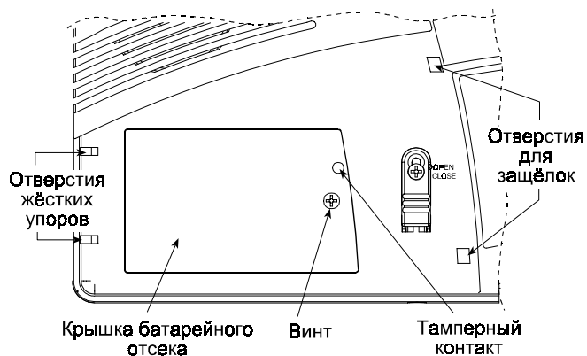
Рисунок 3. Отсек батарей после снятия декоративной крышки
