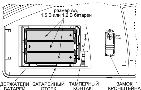
Рисунок 5. Батарейный отсек с установленными батареями
