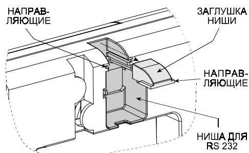
Рисунок 27. Удаление заглушки для установки RS-232
