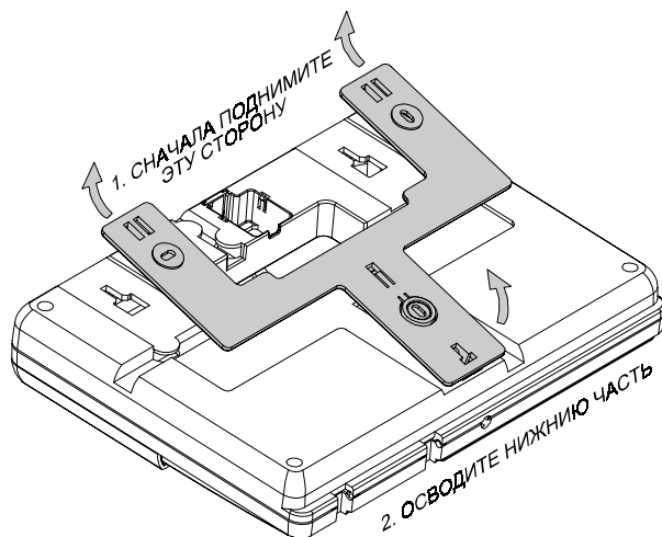
Рисунок 7. Отделение кронштейна
