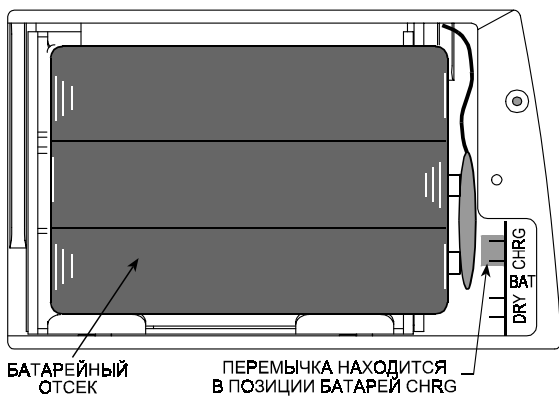
Рисунок 4. Переключатель типа батарей
