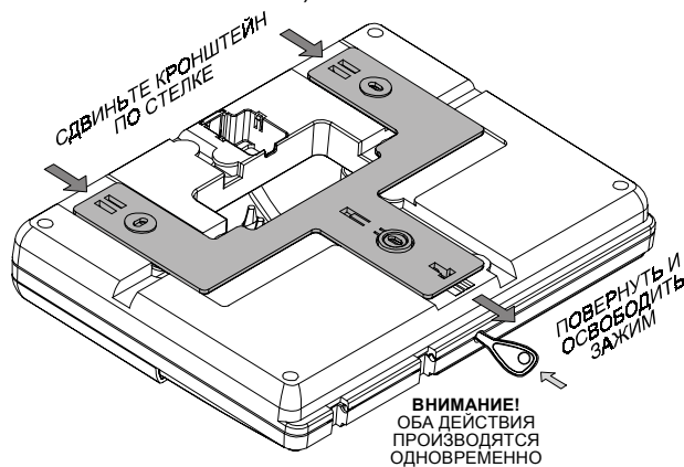
Рисунок 6. Освобождение узкой части кронштейна из зажима.
