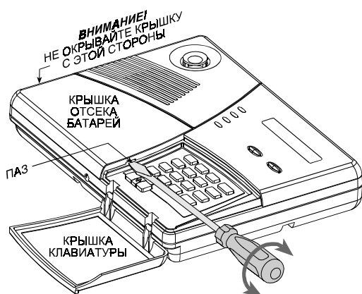
Рисунок 1. Открывание крышки
