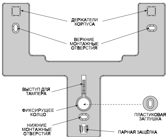
Рисунок 8. Кронштейн - Вид спереди
