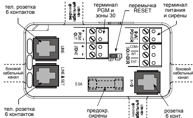
Рисунок 9. Расположение элементов в нише для подключения
