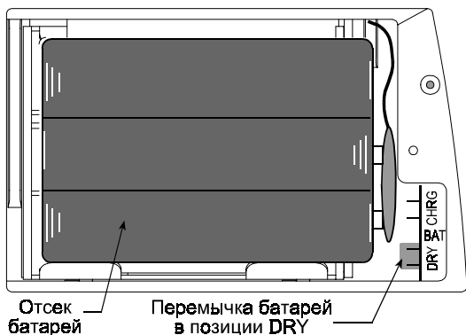
Рисунок 31. Перемычка находится в позиции батарей Dry
