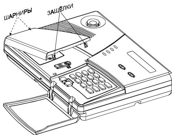
Рисунок 2. Снятие декоративной крышки
