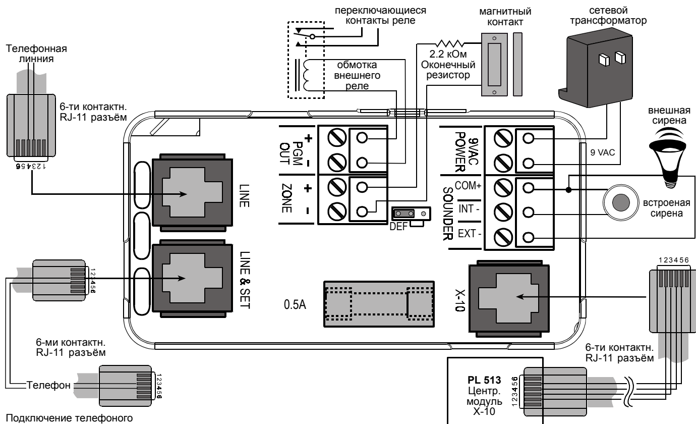
Рисунок 10. Схема подключения
