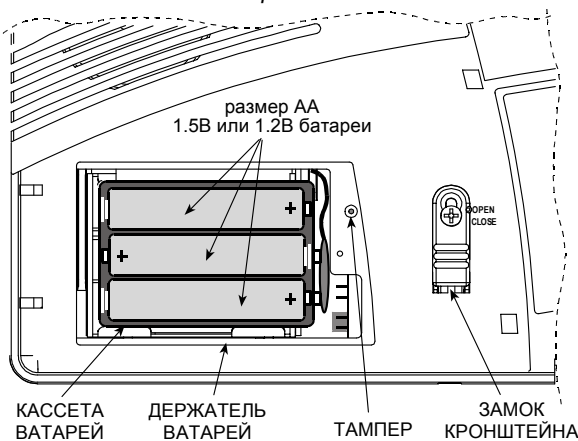
Рисунок 13. Размещение батарей в батарейном отсеке
