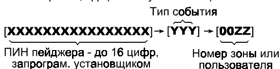
Рисунок 7: Структура сообщения пейджера
