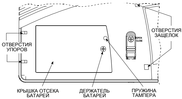
Рисунок 12. Вид батарейного отсека после снятия левой крышки
