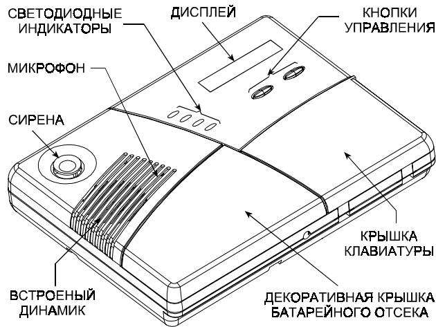
Рисунок 1. Панель управления (с закрытой крышкой)
