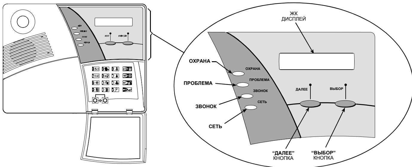
Рисунок 4. Панель управления, кнопки управления и индикаторы
