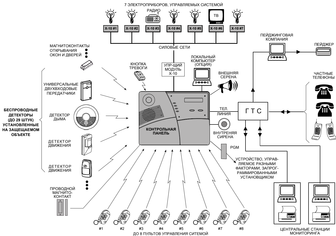
Рисунок 2. Типичная конфигурация системы
