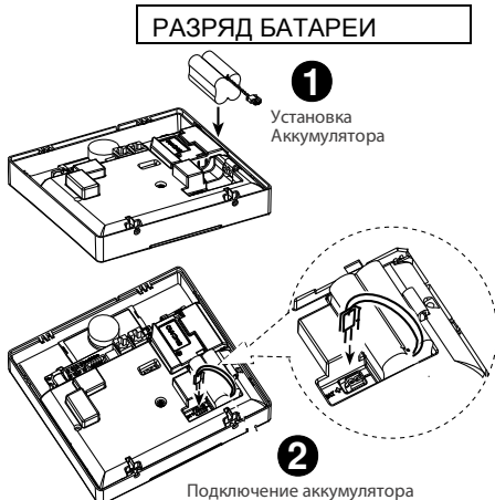
Рисунок 10. Замена аккумулятора
