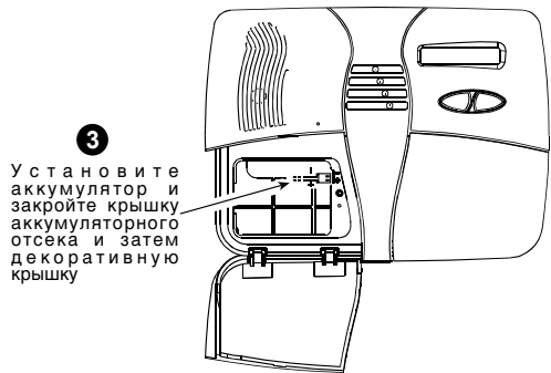
Рисунок 10. Замена аккумулятора
