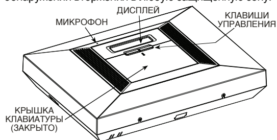
Рисунок 1. Контрольная панель с закрытой крышкой
