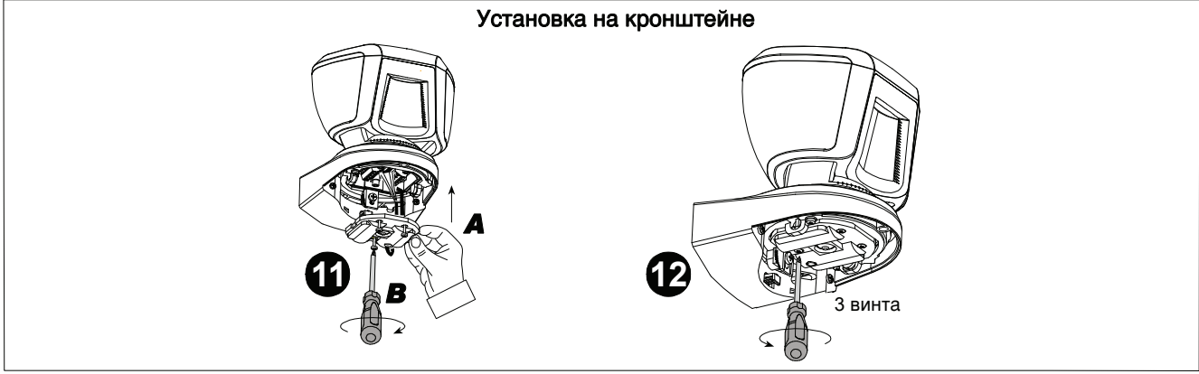
Рисунок 3. Установка.
