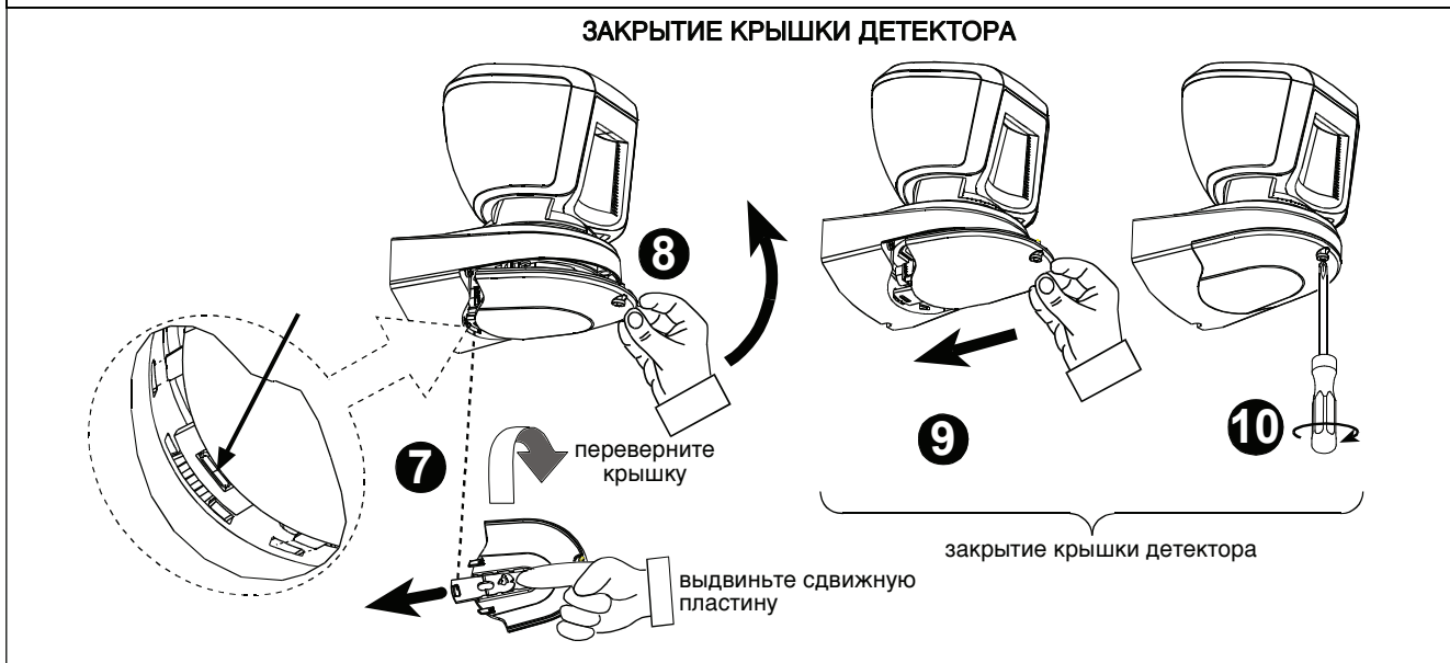
Рисунок 4 Настройка и закрытие/открытие крышки извещателя
