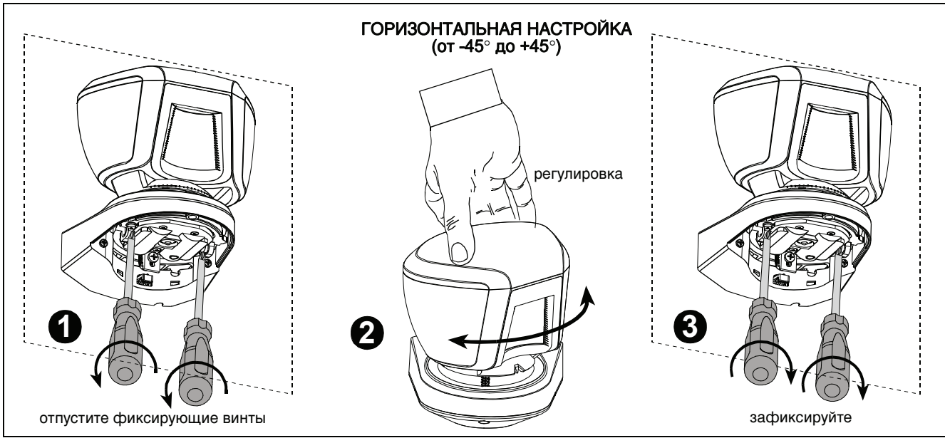
Рисунок 4 Настройка и закрытие/открытие крышки извещателя
