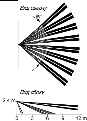
Рис. 2 – Зона обнаружения
